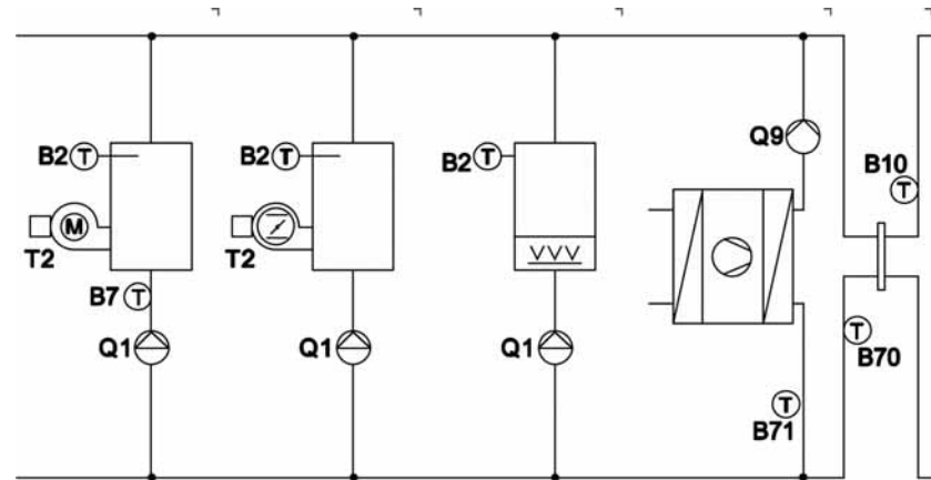
Смешанный каскад RVS43, RVS63, RVS53, RVS41/61
